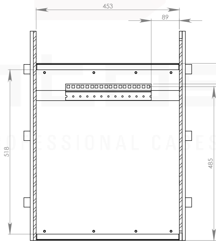
SECTION A-A
