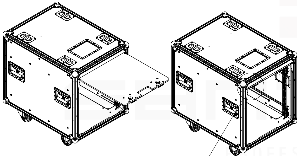
Top sliding door
