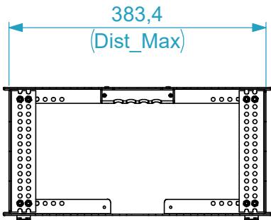
L-L
