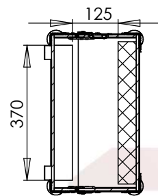
SEÇÃO F-F
