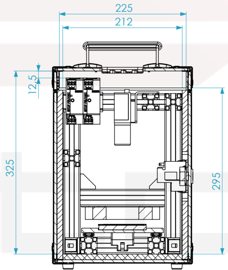
SECTION A-A SCALE 1 : 4
